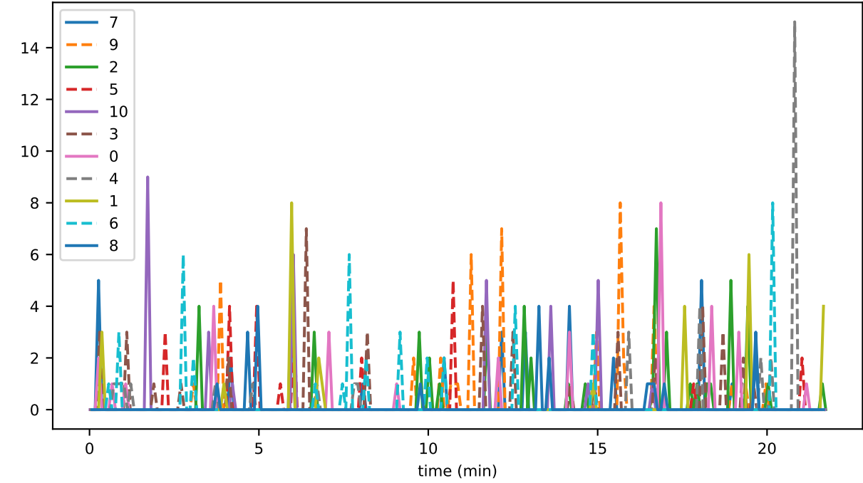
TransactionPrehandler_unhandled_task_count
