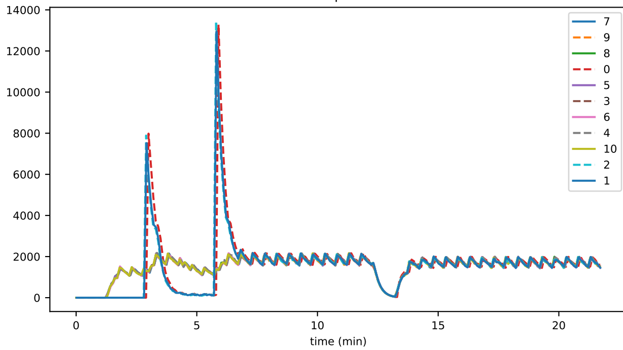
vmUpdate
