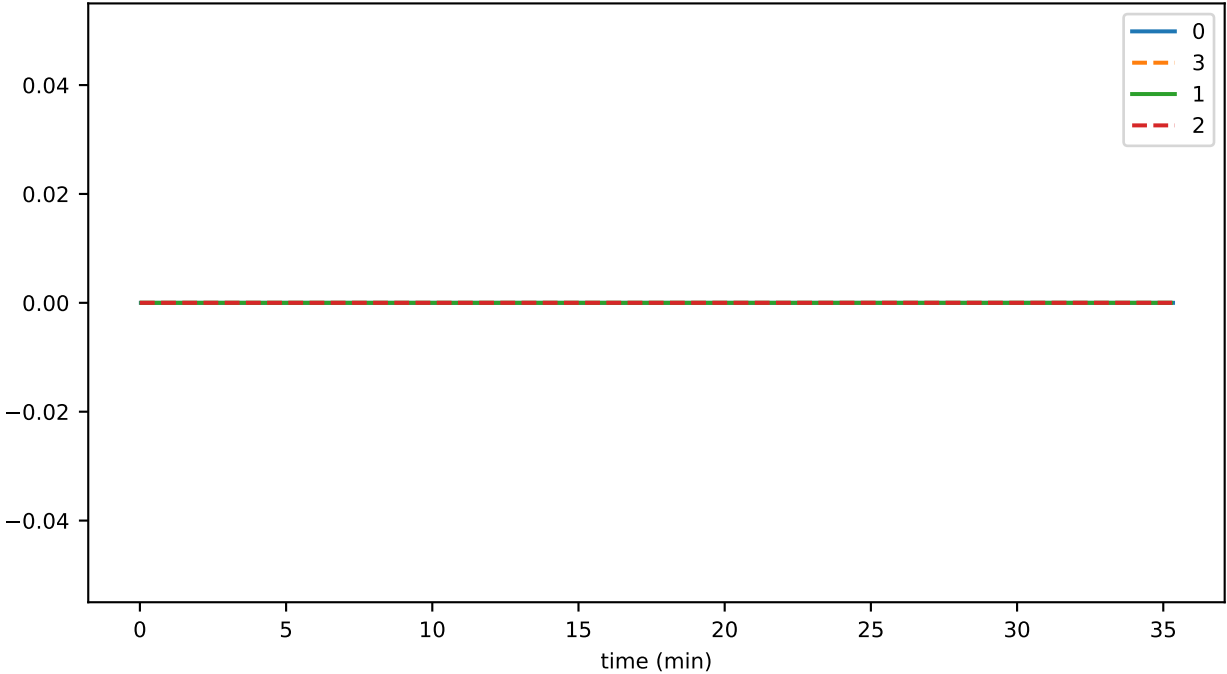
SmartContractService:SystemContractMethodCall_HAS_total
